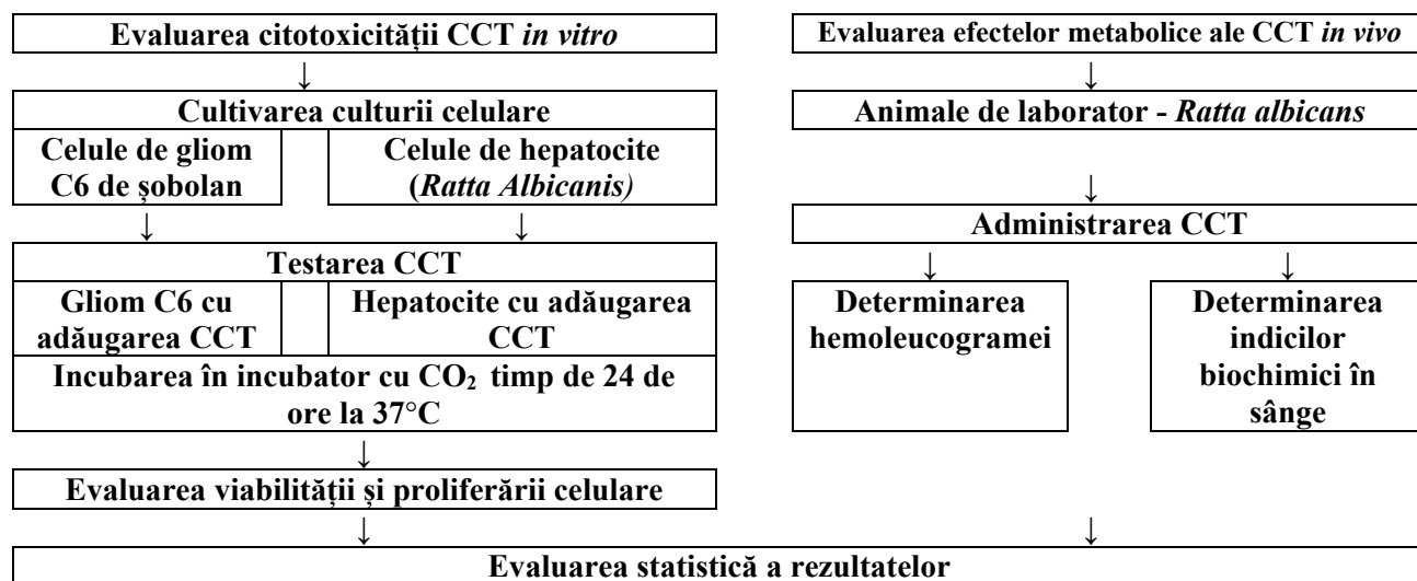
Figura 1. Design-ul studiului
