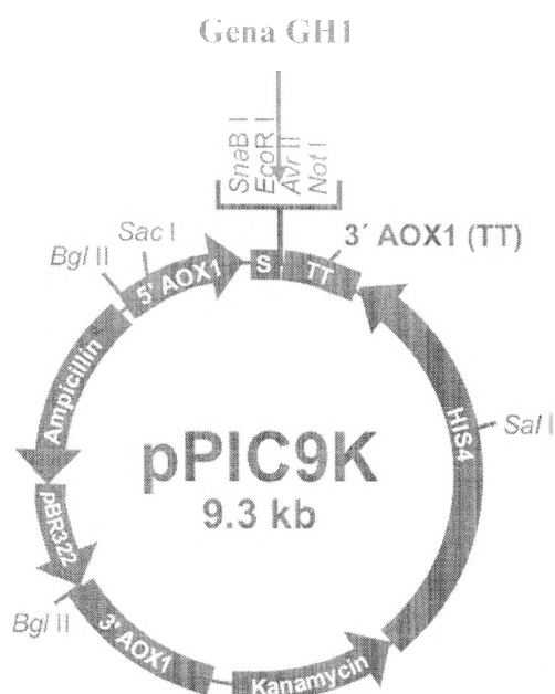
Fig. 1. Reprezentarea grafică a vectorului pPIC9K cu gena GH1 inserată
