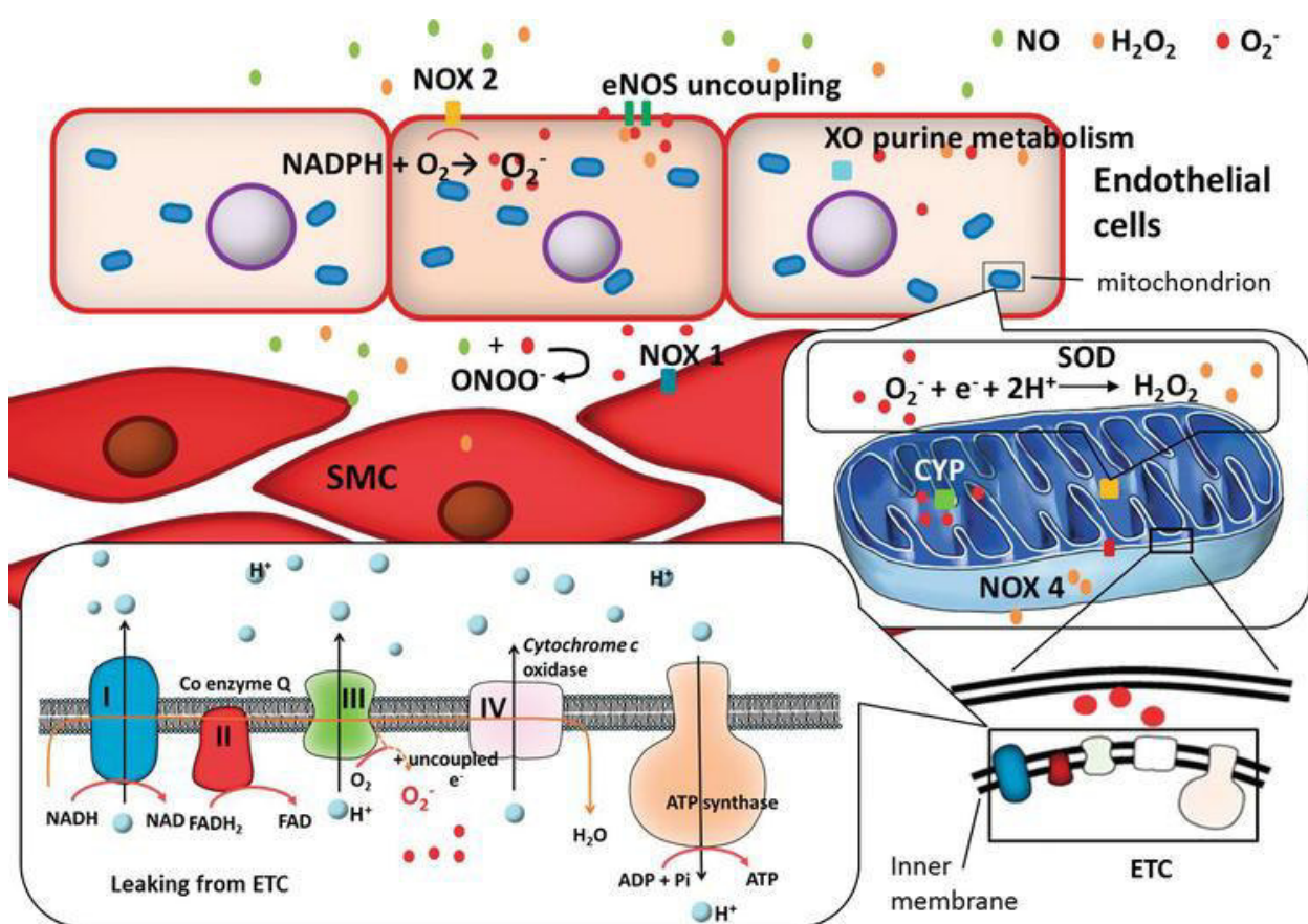
Fig. 1.5. Sursa majoră de specii reactive de oxigen (ROS) și specii nitrogen reactive (RNS) la nivelul țesutului cardiac [după He W., Kwesiga M- P., Gebreyesus E., Liu S. Nitric Oxide and Oxidative
