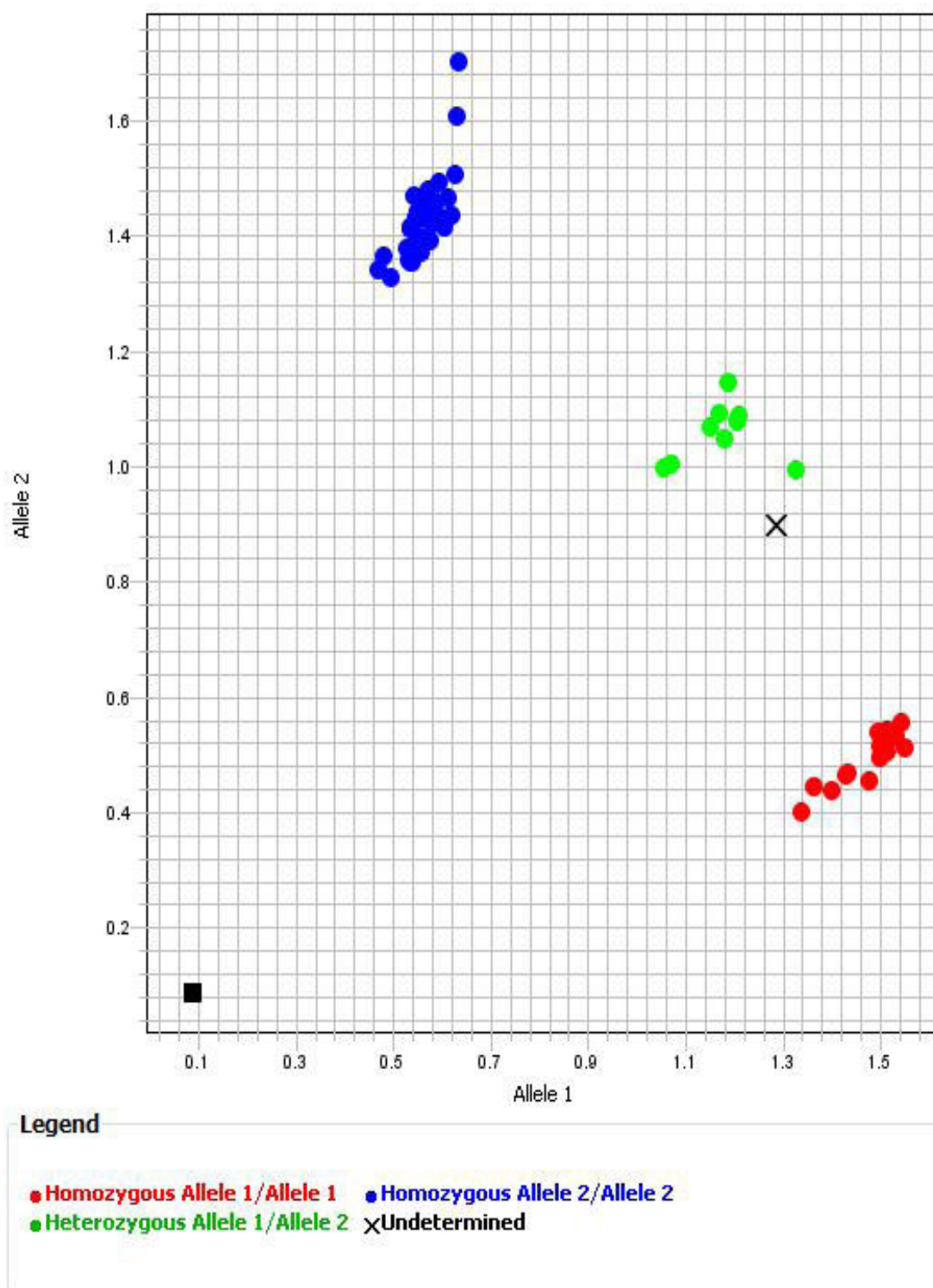
Fig. 5.1. Rezultatele genotipării SNP GJB2_rs80338939 (m.35delG)
