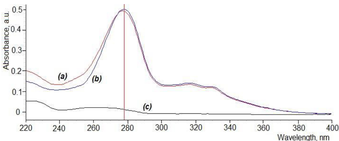
Fig. 3.2. Spectrele de absorbție UV-VIS ale soluției standard de clorhidrat de ciprofloxacina 4,0 \mu\text{g} / ml (a), soluție probă (b) și placebo (c)
