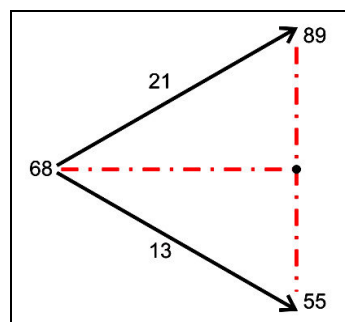
Рис. 21. Пример № 2. Числа ряда Фибоначчи и их деление в соответствии с «Золотой Пропорцией» на «дочерние» отрезки – максимумы 2-го порядка.
