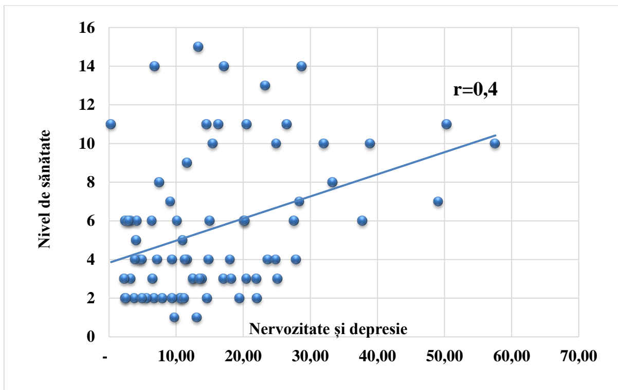
Fig. 4.2. Indicele de corelație a demonstrat o corelație directă a nivelului de înrăutățire a sănătății și nivelului de nervozitate și depresie
